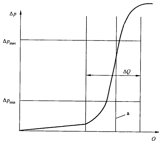
图 A.1 水力特性(图中 a 为设定点流量)
